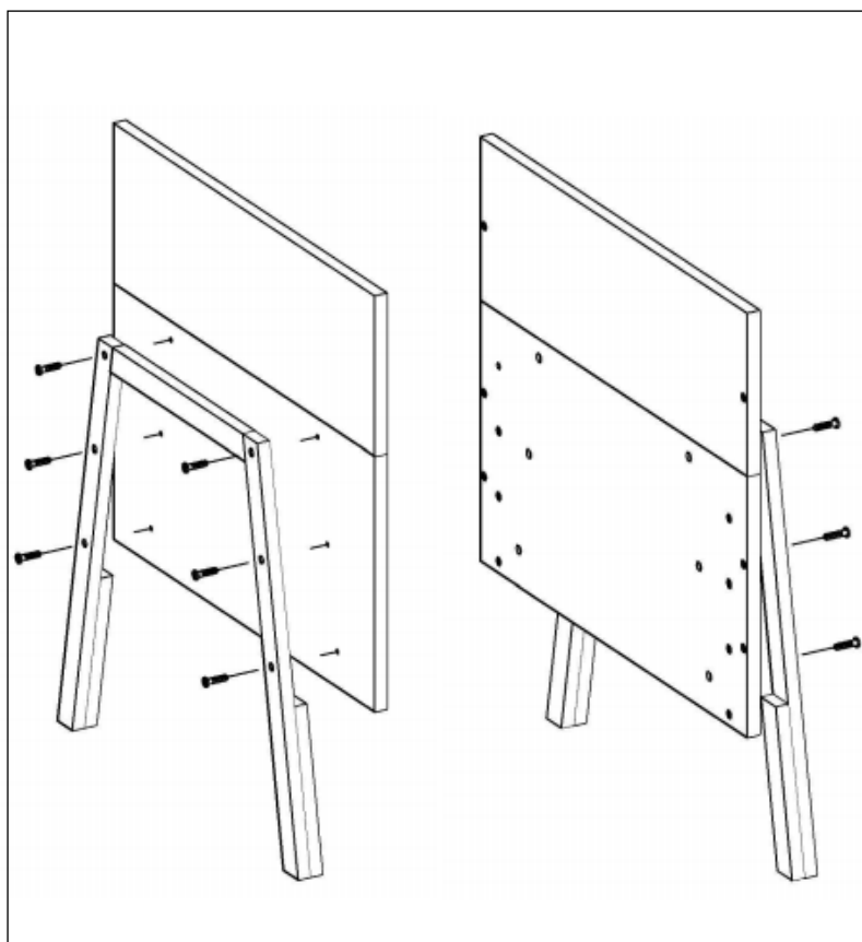
c. M6 x 35 mm Bolt x12
