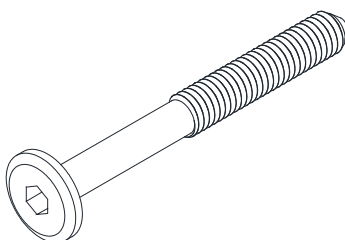
b. M6 x 55 mm בורג x8
