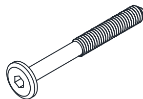
b. בורג M6 x 55 mm x 8
